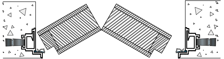
Versione LIBRO A SPINGERE
