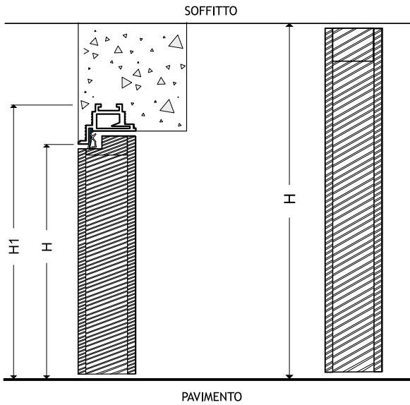
Versione con TRAVERSO SUPERIORE
